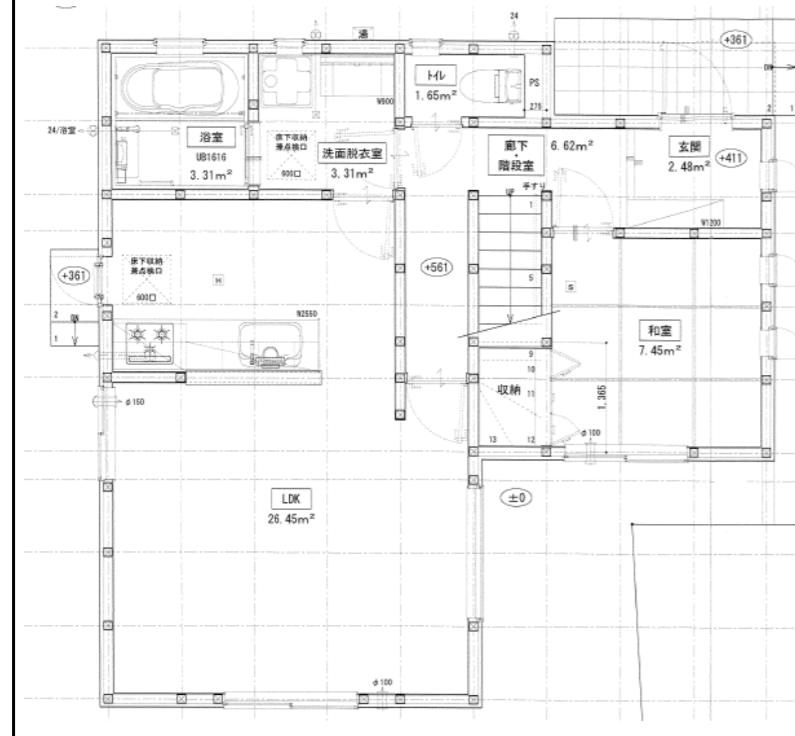
HDIタウンA棟：間取り
